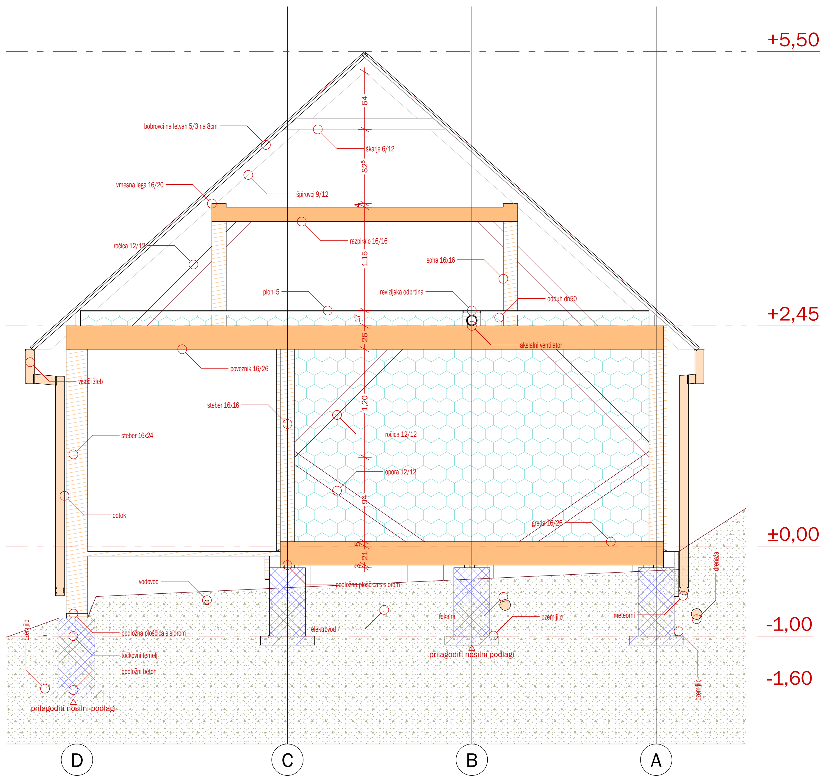
P-4-4 ogrođje os 4 1:25
