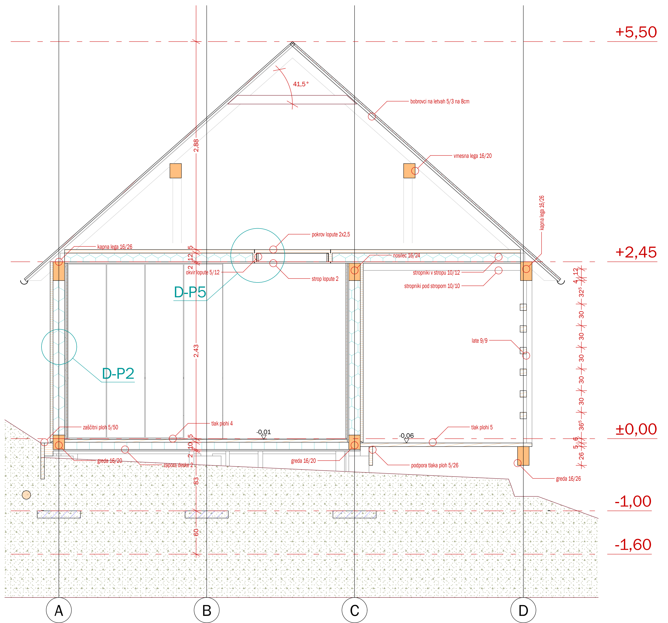
P-2-3 precno os 2-3 1:25
