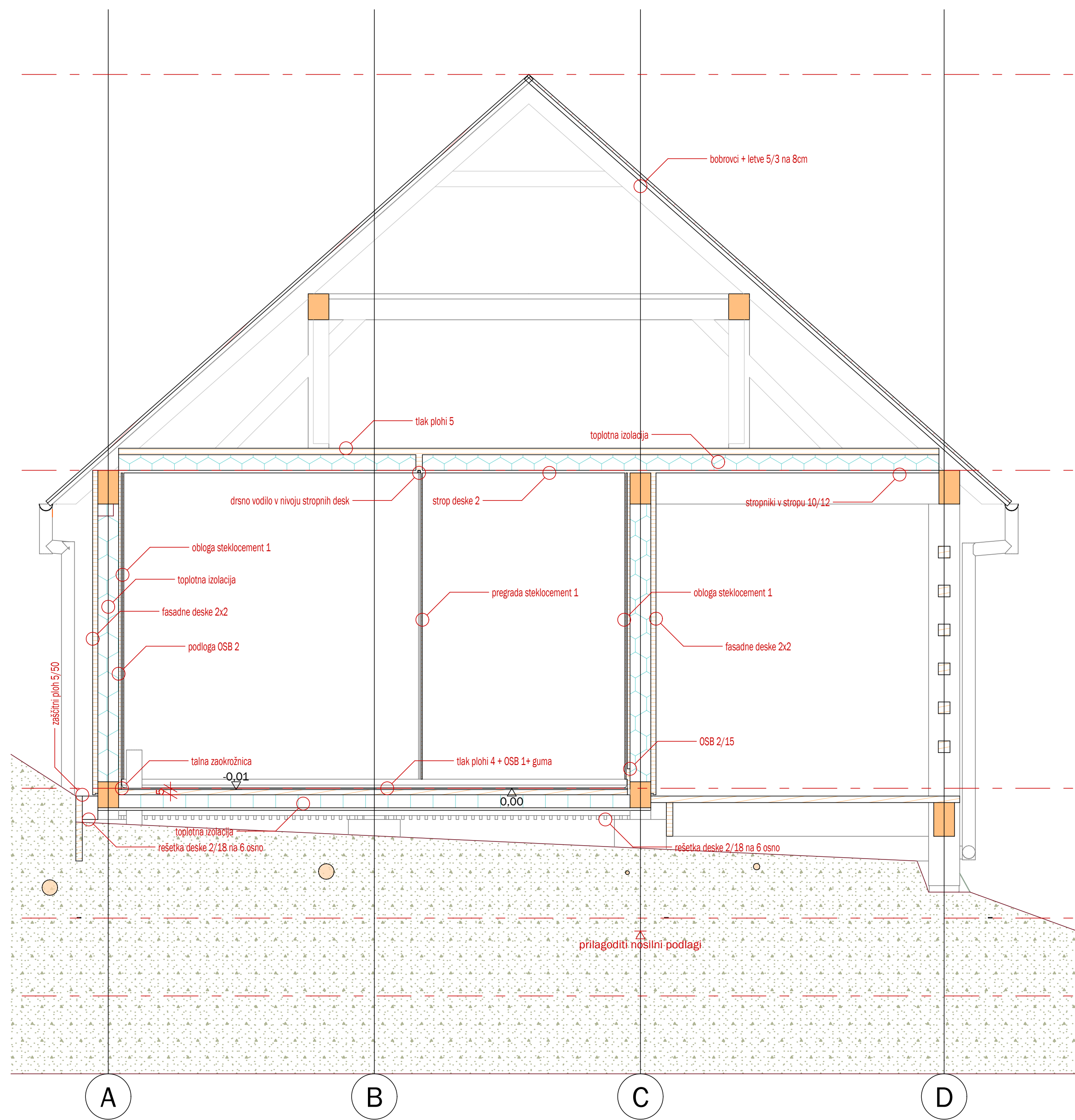
P-3-4 precno os 3-4 1:25
