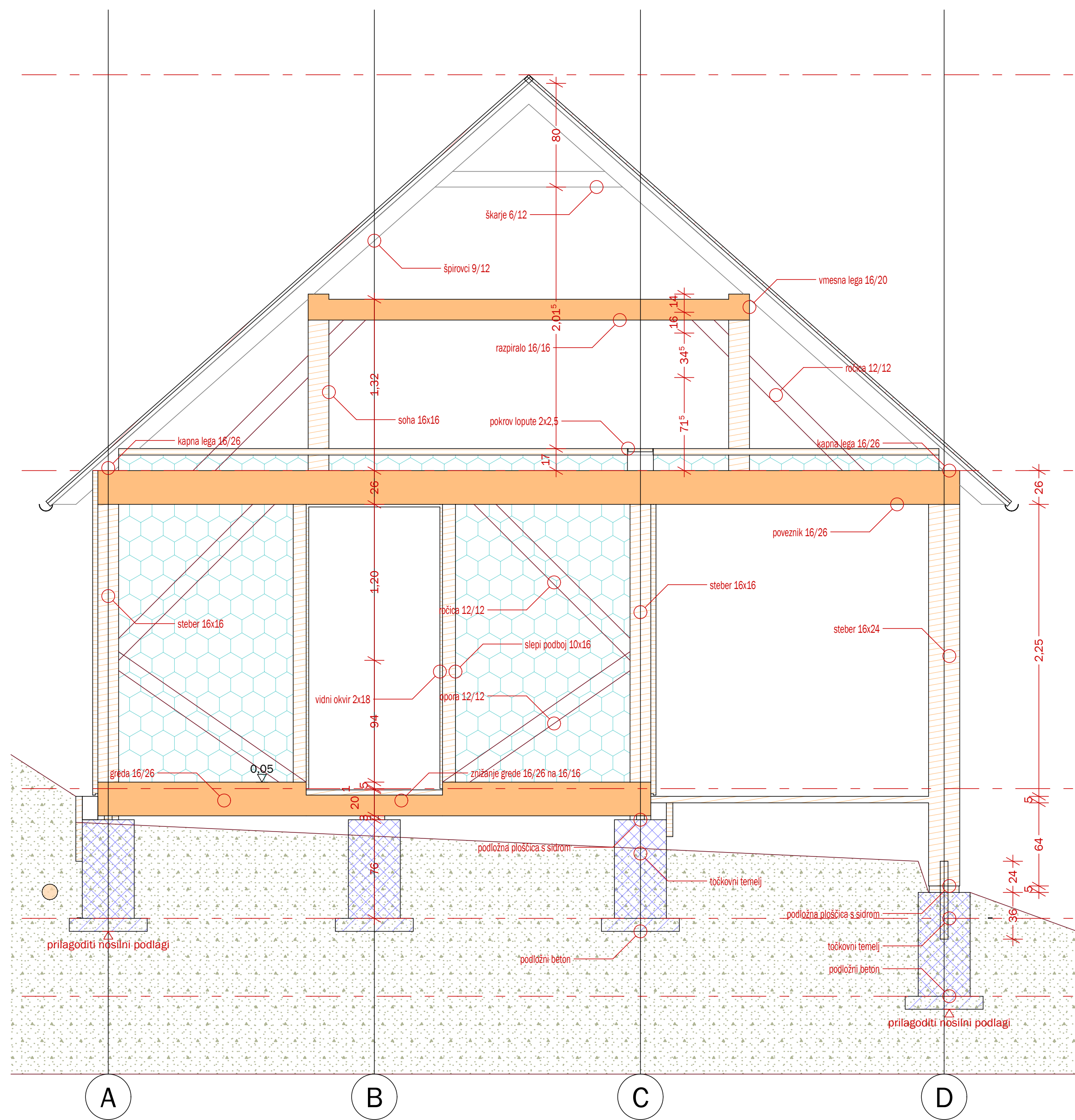
P-1-1 ogrođje os 1 1:25
